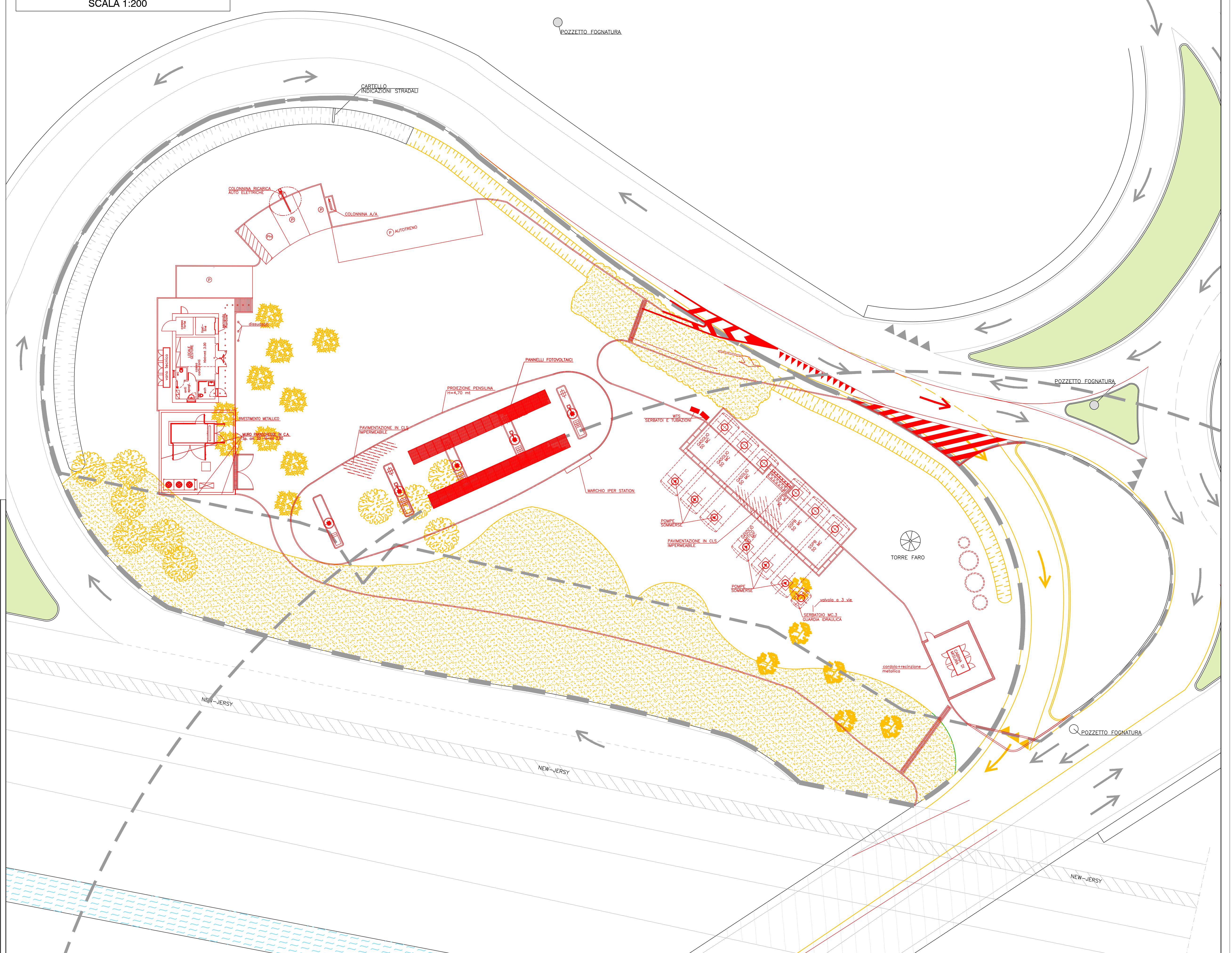
PLANIMETRIA STATO DI SOVRAPPOSIZIONE SCALA 1:200
